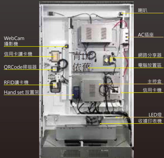
門板內部
