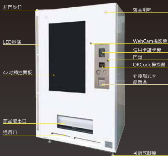
外觀正面
