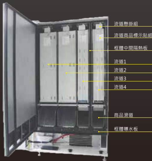
機台內部
